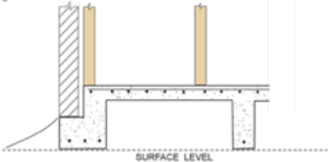
Fig 2 Waffle Slab
